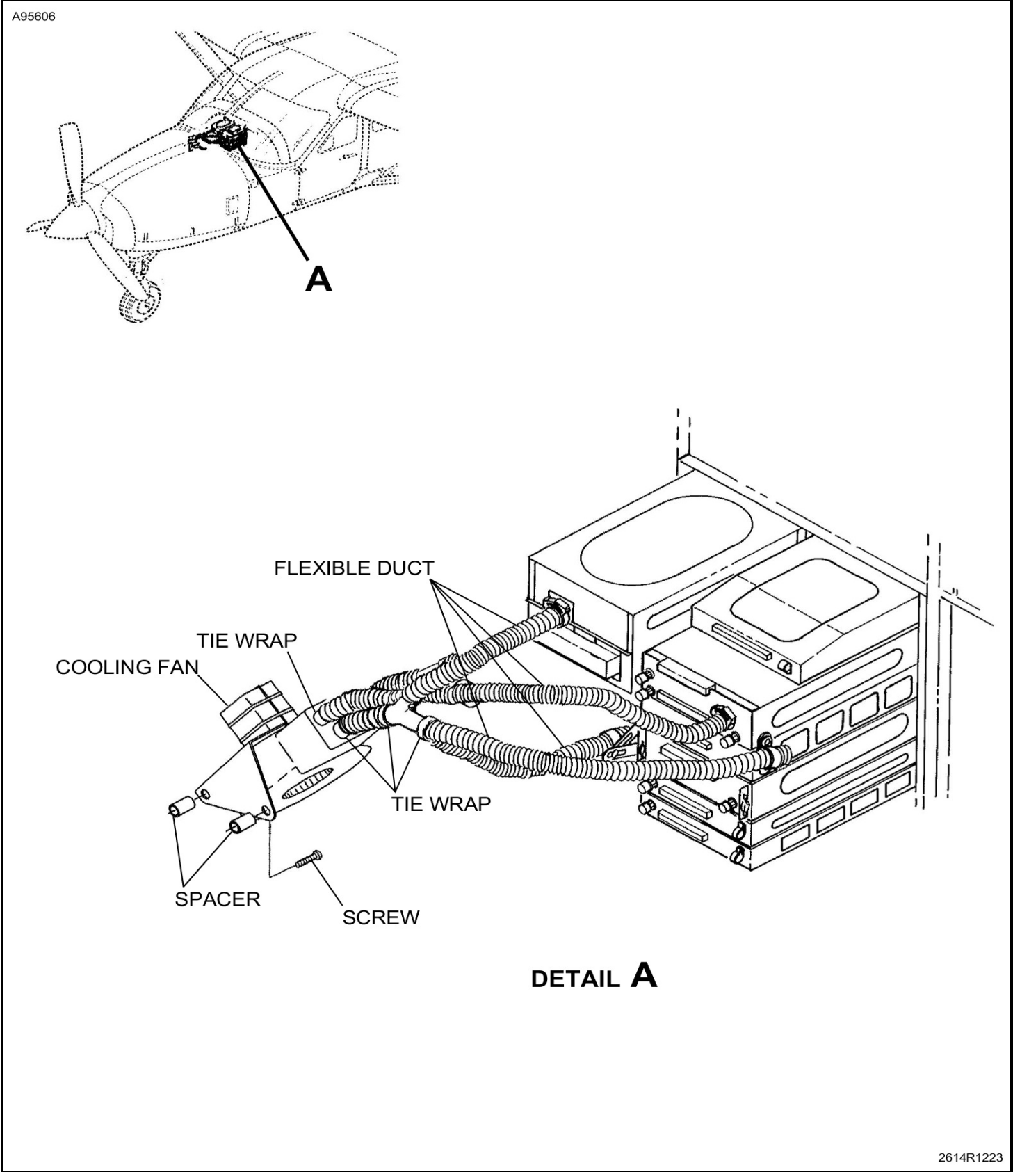
Figure 401 : Sheet 1 : Avionics Cooling Fan
